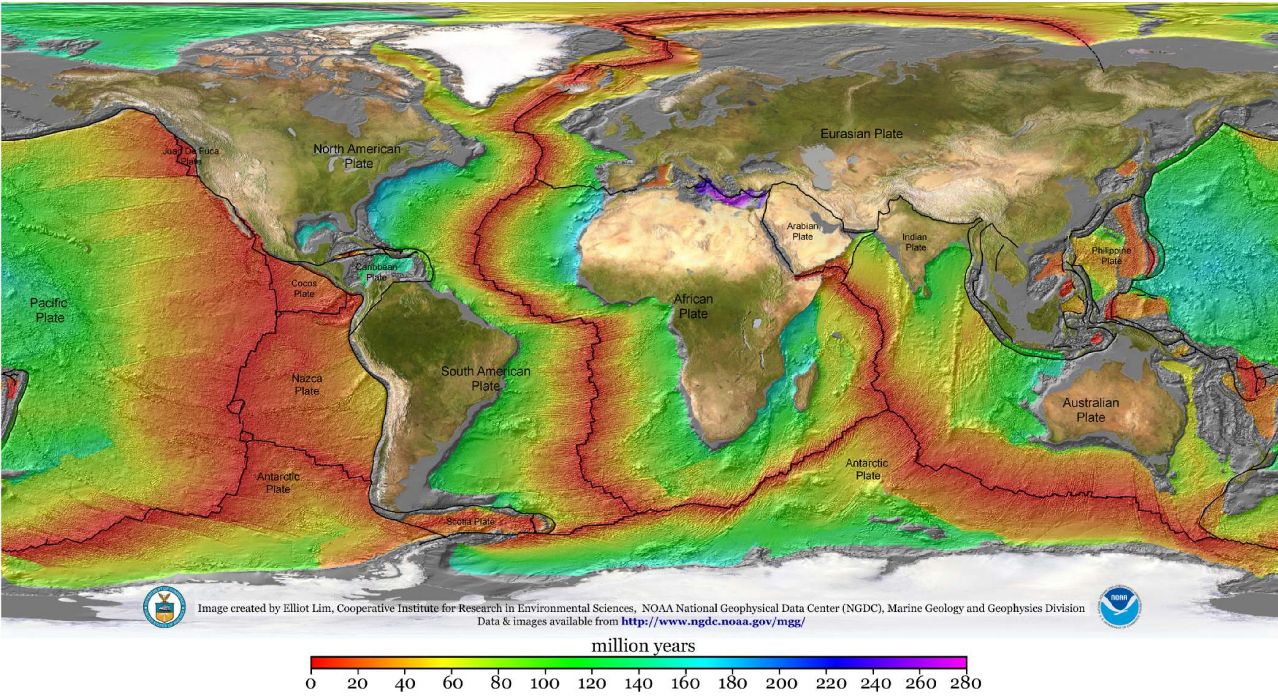
Età della litosfera oceanica (Ma)
